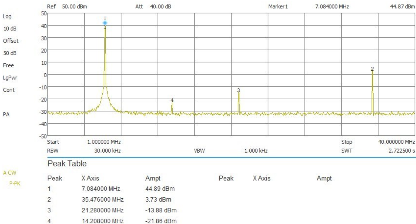
Abbildung 9 – Oberwellen 40m bei 5W-Steuerleistung
