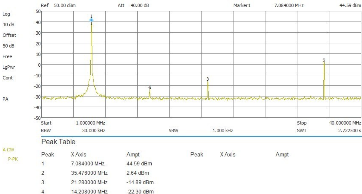
Abbildung 8 – Oberwellen 40m bei 4W-Steuerleistung
