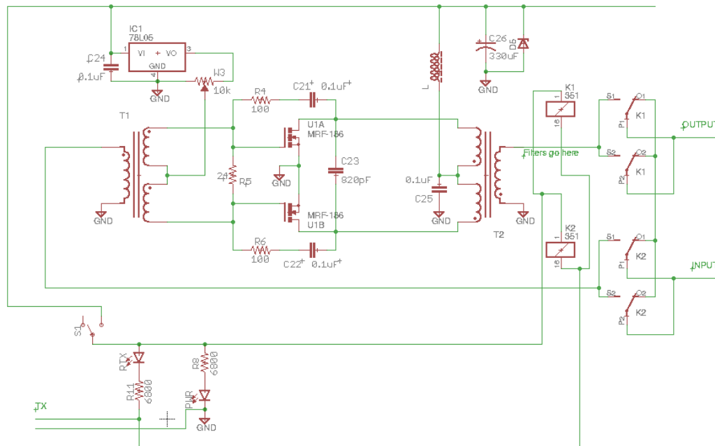
Abbildung 39 – Unvollständiges Schaltbild der Endstufe
