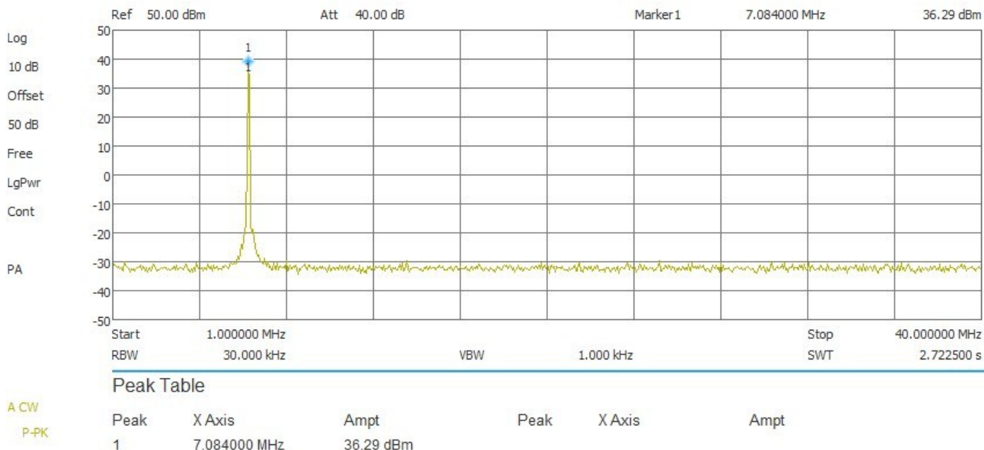
Abbildung 4 – Oberwellen 40m bei 5W des IC-705
