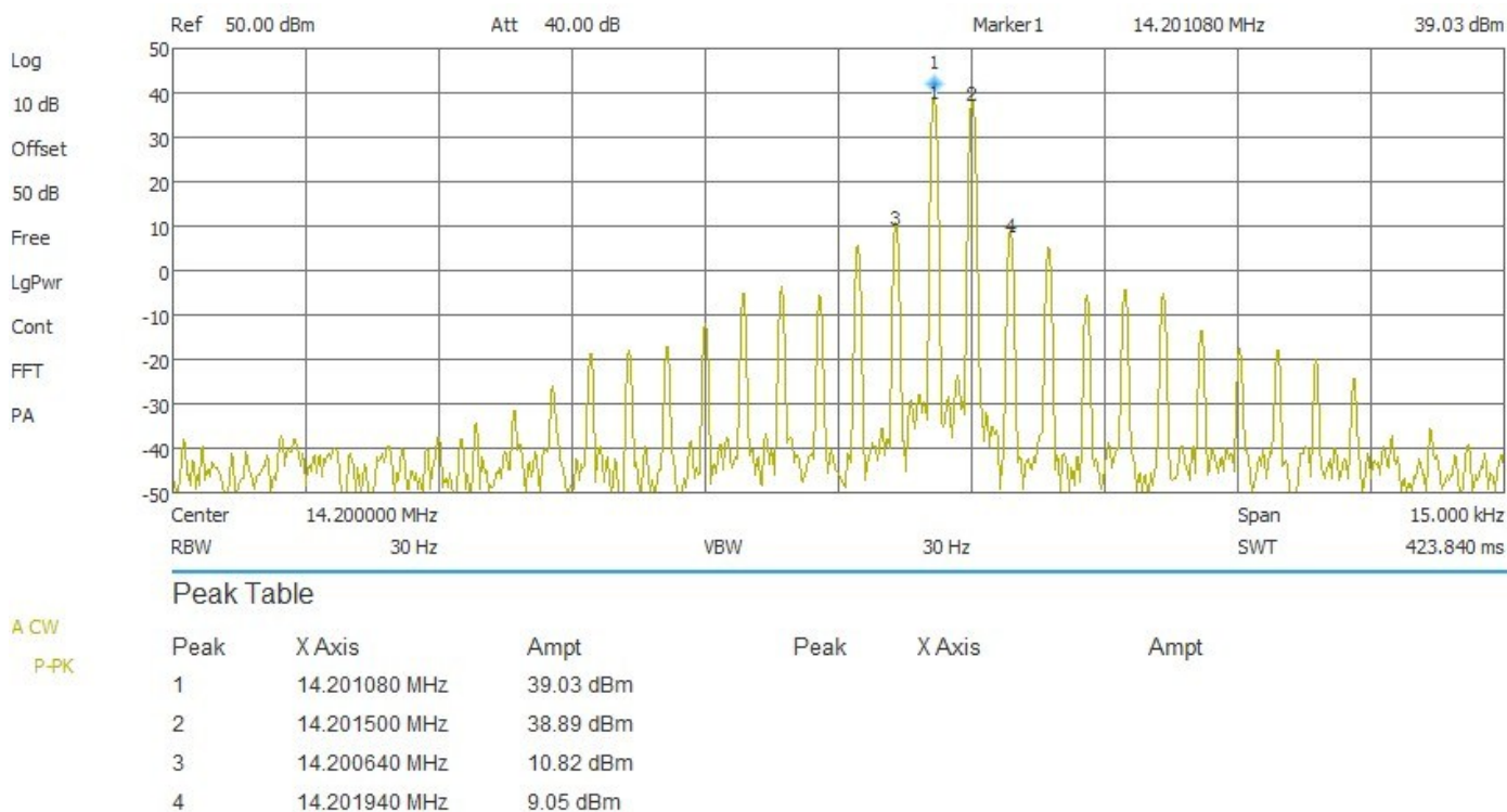
Abbildung 21 – Spektrum IM 3 PA bei 3W Steuerleistung
