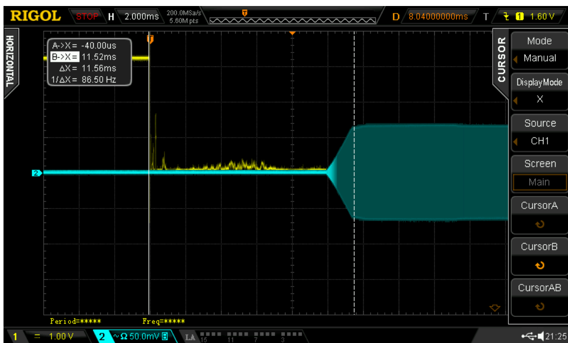
Abbildung 35 - Tastzeit IC-705
