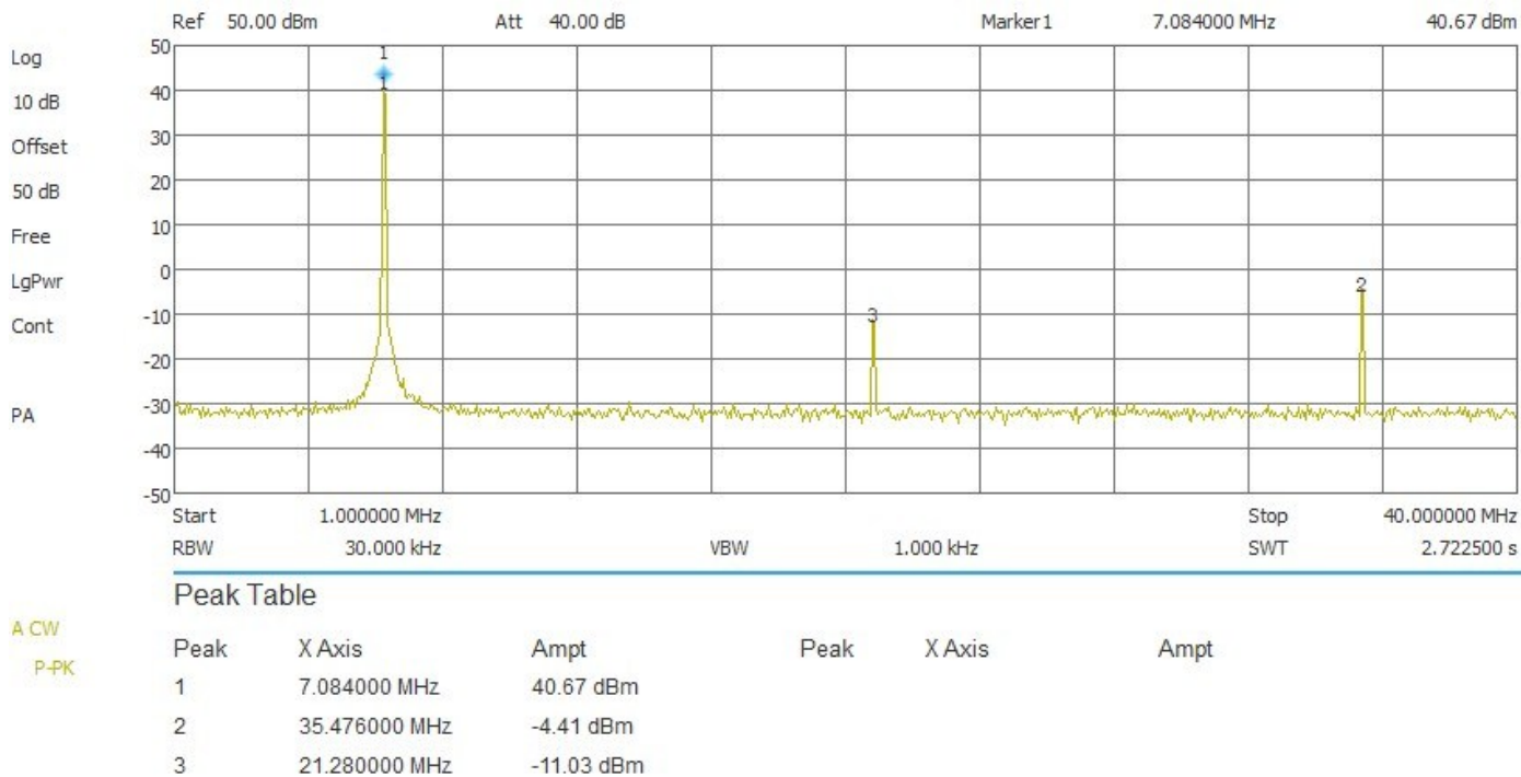
Abbildung 5 – Oberwellen 40m bei 1W-Steuerleistung
